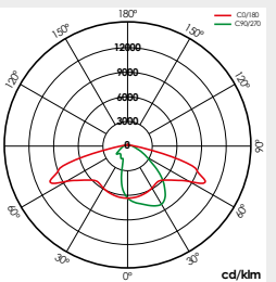
VA02L0M (≤700mA) 80Led
