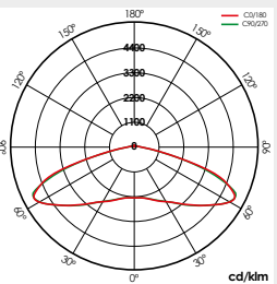
SI50L0M (≤700mA) 80Led
